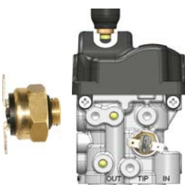
Segnalatore elettrico di pressione. Pressure signal assembly
